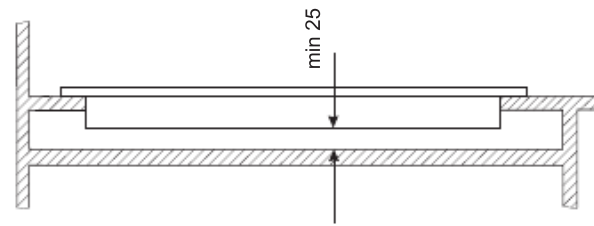
Installera spishäll i köksskåp
