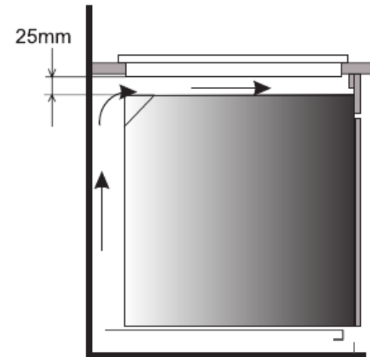
Installera spishäll i köksbänk ovanför ugn med ventilation.
